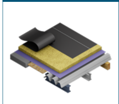
Flachdach mit Dichtungsbahn | siehe Seite 208
