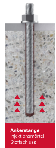
Betonschraube Hinterschnitt Formschluss
