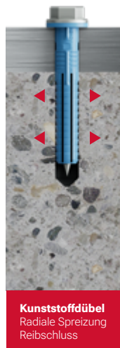
Kunststoffdübel Radiale Spreizung Reibschluss
